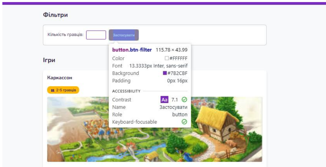
Рис. 6 — Перевірка контрастності елементів за допомогою DevTools
